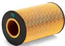
H= 206mm OD= 119mm ID=54 mm ID2=137 mm / 129 mm
